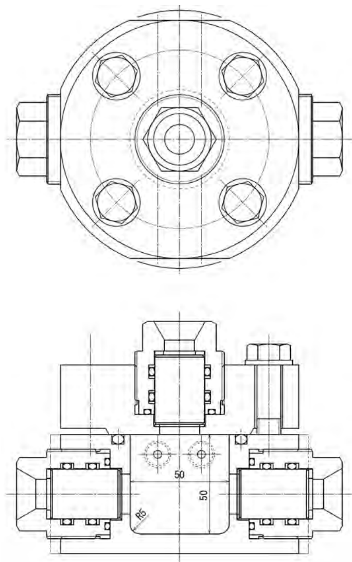
可視窓付き高圧セル断面図
